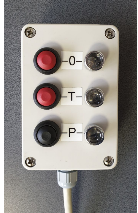
Bedienbox 6 Funktionen Nullstellen/Brutto 0, Tariieren/Netto 0, Drucken/Druckkontrolle
