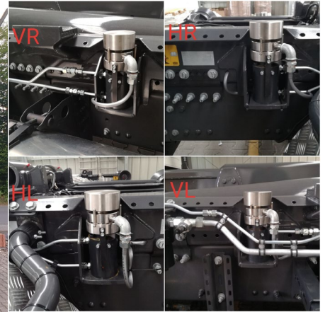
Wägemechanik
